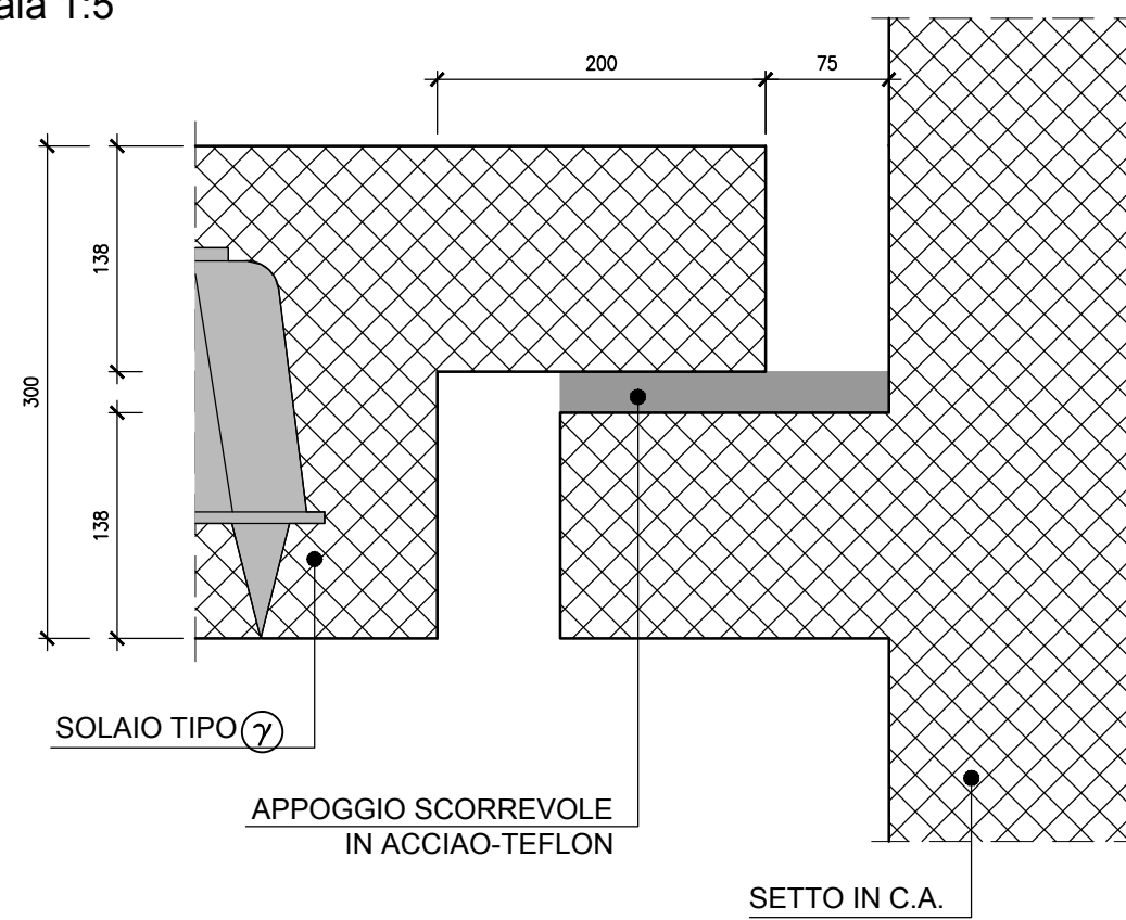
DETTAGLIO TIPICO GIUNTO STRUTTURALE SEZIONE 3-3 Scala 1:5
